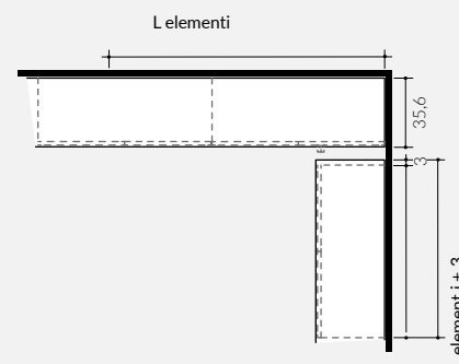
Top e controtop per mobile ad angolo Dx
