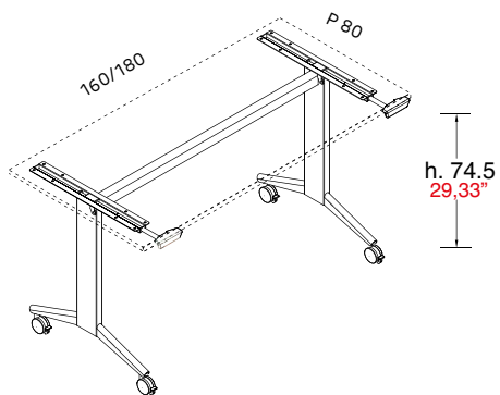
Tavolo con ruote frenanti e piano ribaltabile flip
