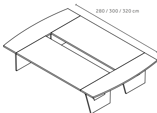
Composizione tavolo riunioni con top lineari
