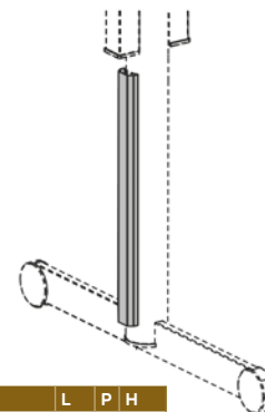
Canale passacavi verticale per gamba intermedia H. 40
