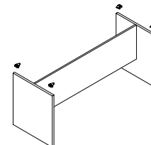
Struttura PANEL in melaminico
