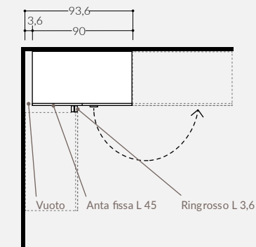
Mobile ad angolo Dx
