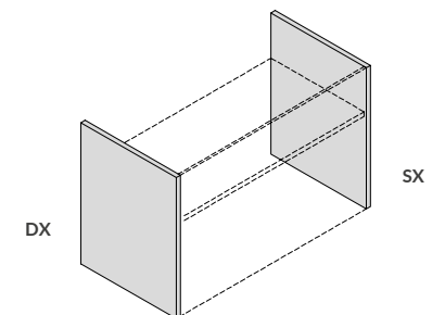
Fianchi finali sp cm 33,5 H cm 105,5
