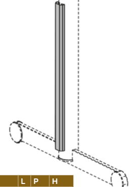
Canale passacavi verticale per gamba terminale H. 55
