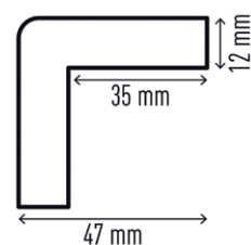
art. 1102 - Profilo paracolpi angolare C35
