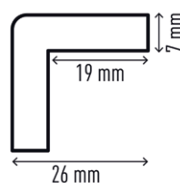
art. 1101 - Profilo paracolpi angolare C19
