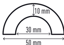
art. 1115 - Profilo paracolpi per tubolari P30
