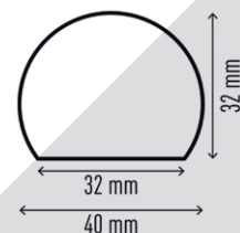
art. 1109 - Profilo paracolpi per superfici S32R
