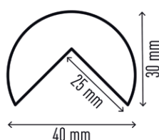
art. 1100 - Profilo paracolpi angolare C25R
