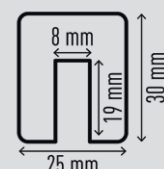
art. 1127 - Profilo paracolpi per spigoli E8
