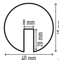
art. 1126 - Profilo paracolpi per spigoli E8R
